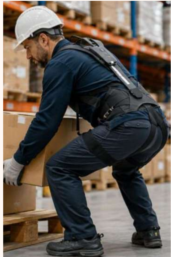
Exoesqueleto pasivo
